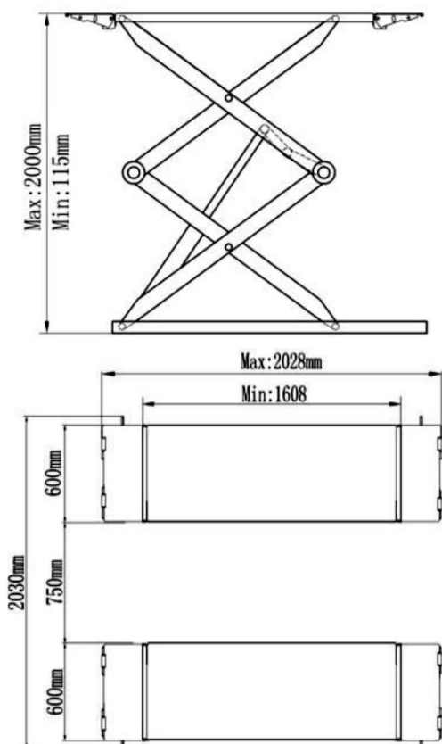
* podwójny system podnoszenia (2 siłowniki)
